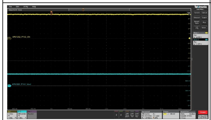
Fig. 13: AP61302Z6-7 _P1V2_Vin Vout
